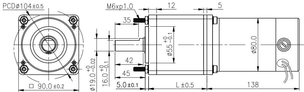
外形尺寸/ Appearance Size
