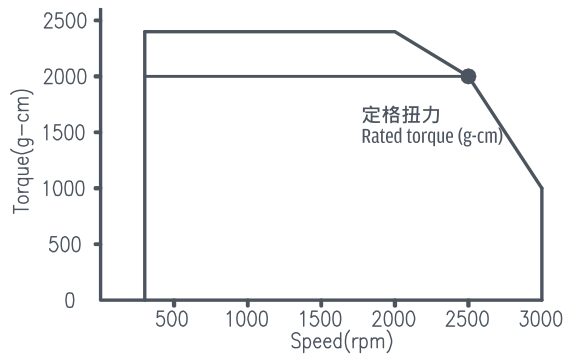
馬達單體特性/ Motor Characteristics
