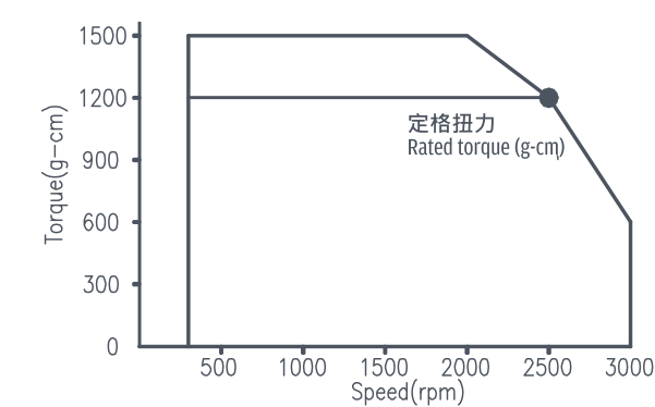
馬達單體特性/ Motor Characteristics
