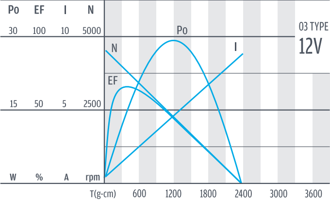
馬達單體特性/ Motor Characteristics
