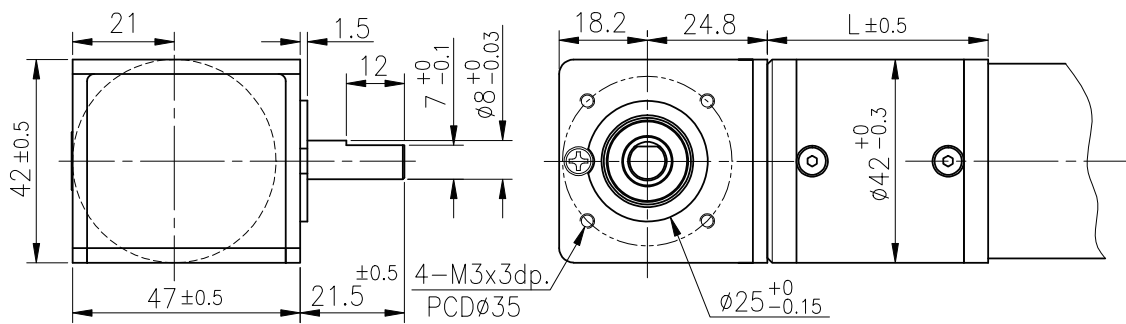
外形尺寸/ Appearance Size
