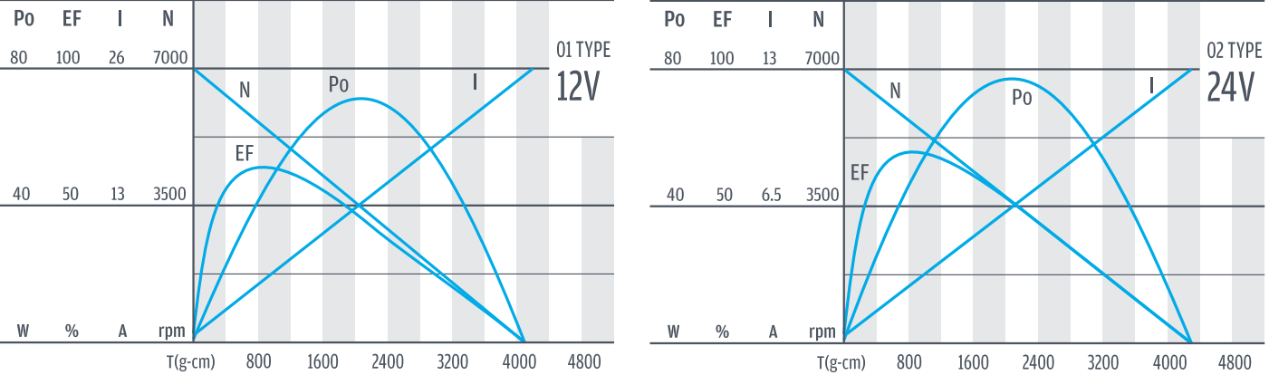
馬達單體特性/ Motor Characteristics
