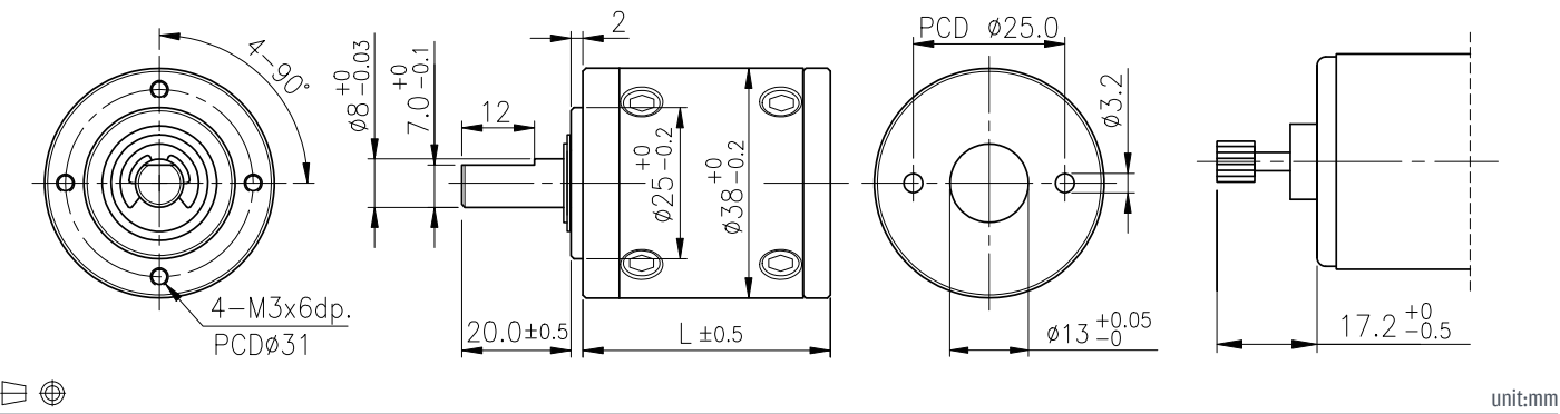
外形尺寸 & 馬達裝卸方法/ Appearance Size & Motor Installation
