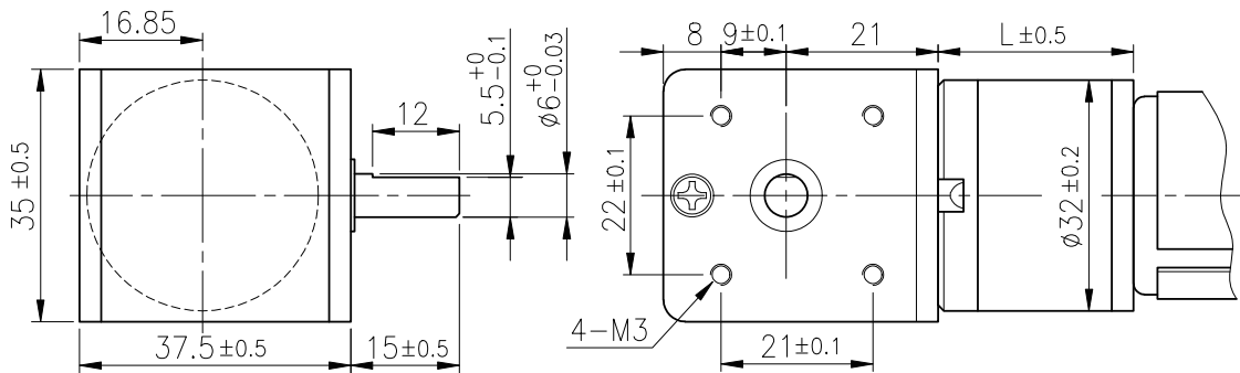
外形尺寸/ Appearance Size
