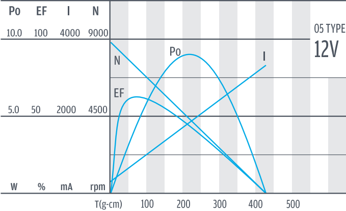
馬達單體特性/ Motor Characteristics
