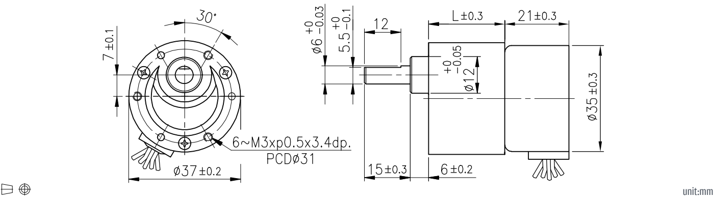
馬達單體型式/ Motor Data
