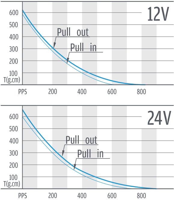
馬達單體特性/ Motor Characteristics
