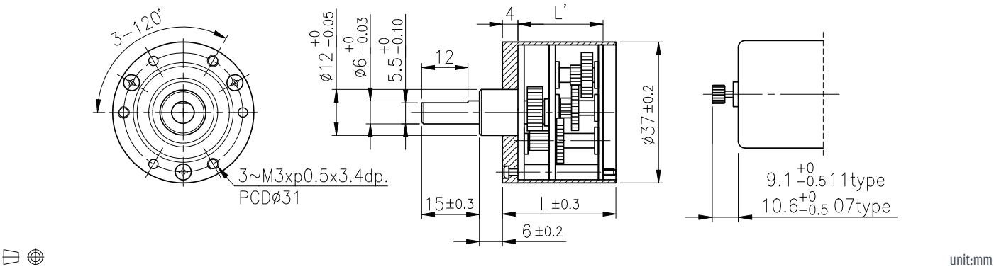
外形尺寸 & 馬達裝卸方法/ Appearance Size & Motor Installation
